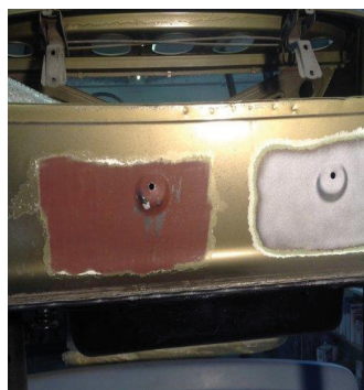
Décapage de peinture – vieille voiture (oldtimer): à gauche : seulement avec de la glace carbonique – à droite: avec un mélange de glace carboglace et d'abrasif
